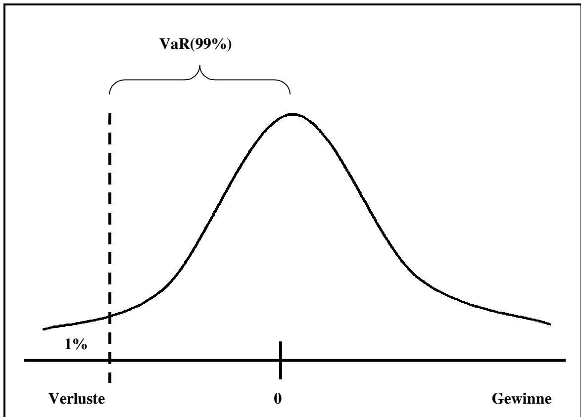
Abb. 1: Value at Risk für ein Konfidenzniveau von 99%
