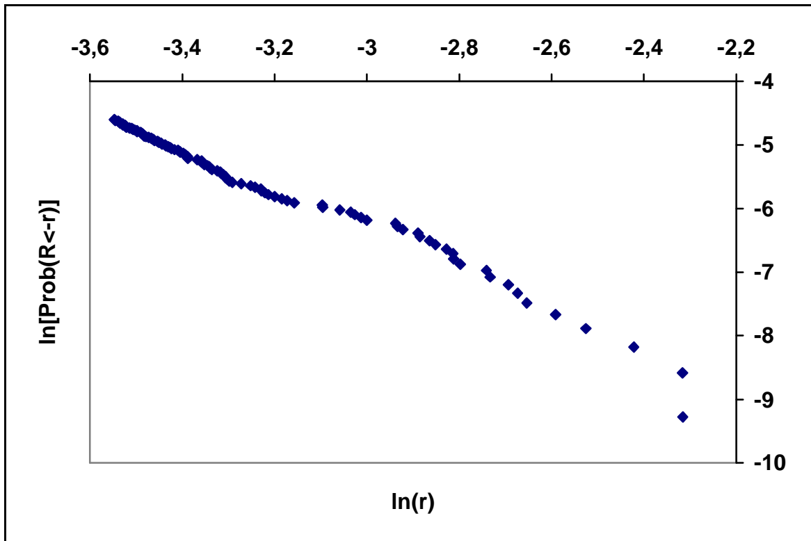
Abb. 2: Doppelt logarithmische Darstellung der kumulierten Häufigkeitsverteilung von Dax-Tagesrenditen (30.9.1959 – 5.7.2002)
